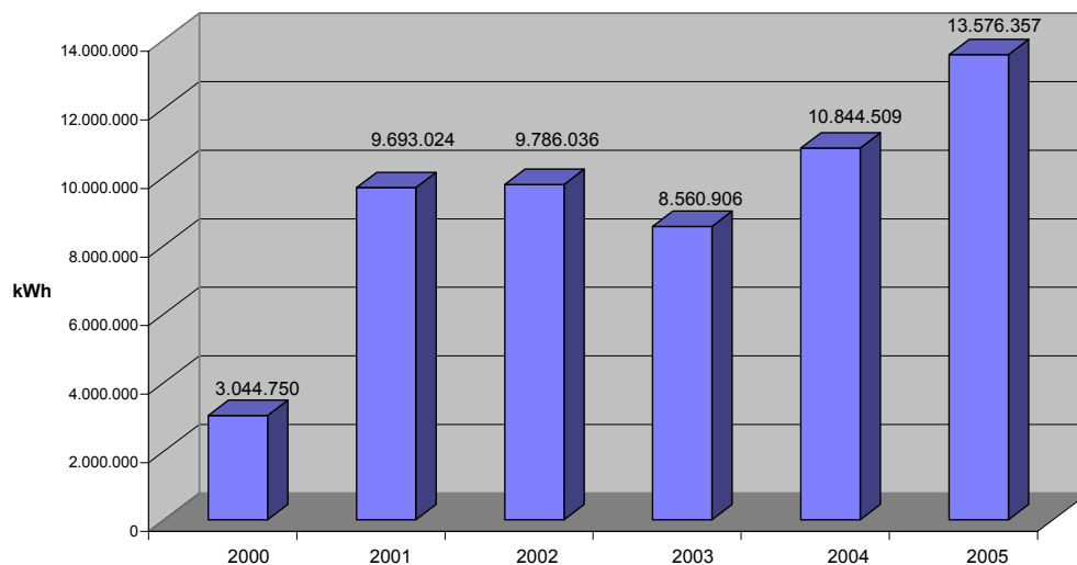
Raforkuvinnsla í Orkustöð 2000-2005
