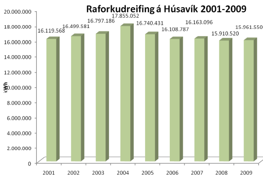
Mynd 3: Innmötun til Húsavíkur árin 2001 til 2008, mæld í kWh
